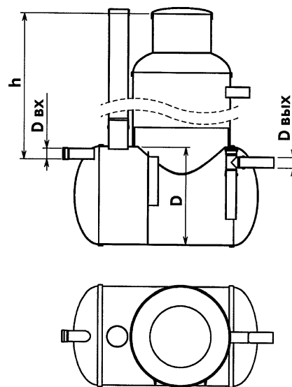
Горизонтальный жиросепаратор
