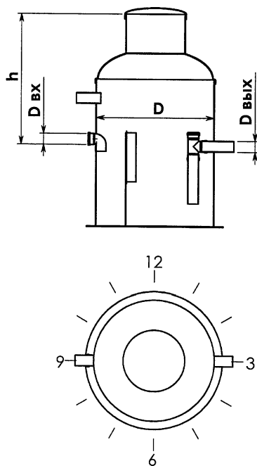
Вертикальный жиросепаратор
