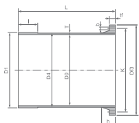
втулка «гладкий конец - фиксированный фланец»
