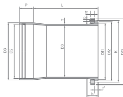
втулка «раструб - фиксированный фланец»
