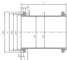
втулка «раструб - свободный фланец»
