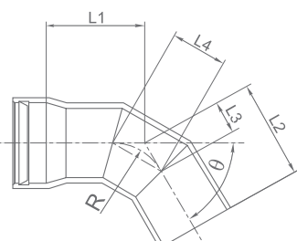
Отвод 60°
