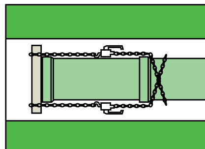
Соединение труб HELYX
