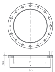
фланец свободный стеклопластиковый
