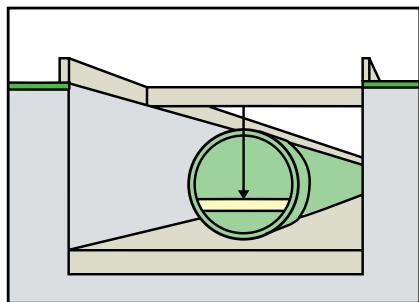
Центровка трубы
