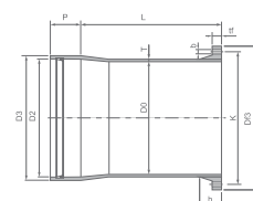
втулка «раструб - фиксированный фланец»
