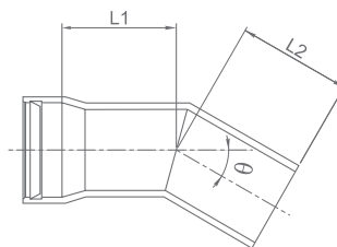
Отвод 30°
