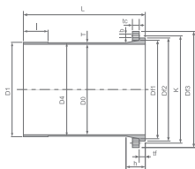
втулка «гладкий конец - фиксированный фланец»
